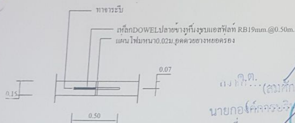
รูปขยาย EXPANSION JOINT
