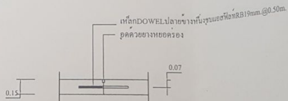
รูปขยาย CONTRACTION JOINT
