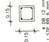
ขยาย C1 มาตราส่วน 1:25
